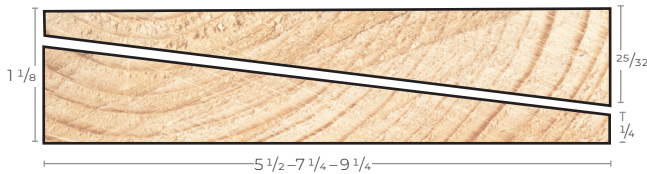
5/4 BEVEL SIDING N° 8A
