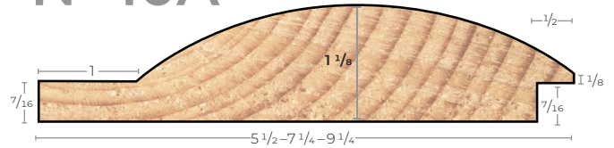
5/4 LOG SIDING N° 10A
